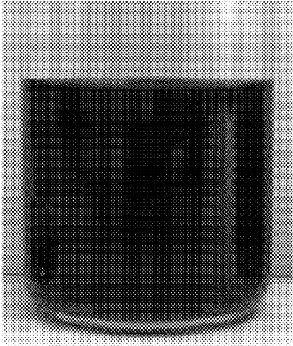
(A). Ethanol
